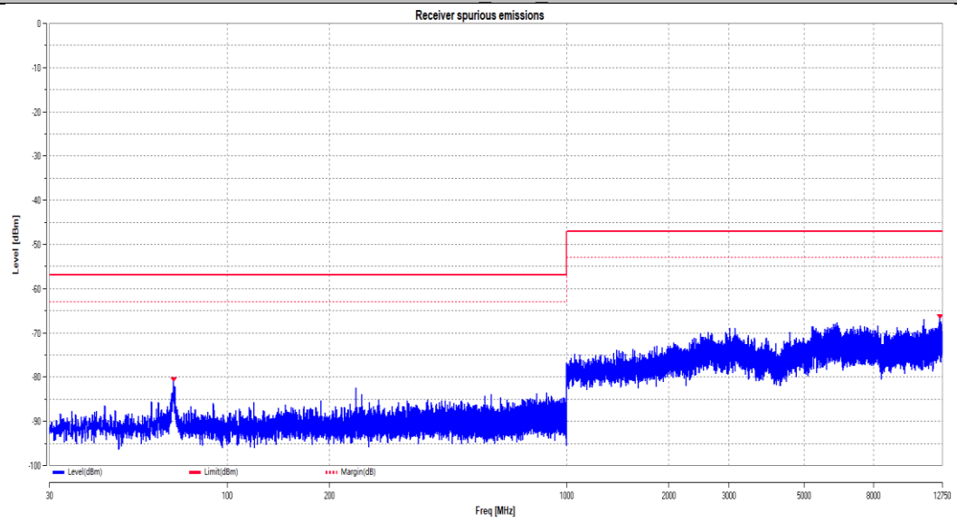
11N40SISO Ant1 2462
