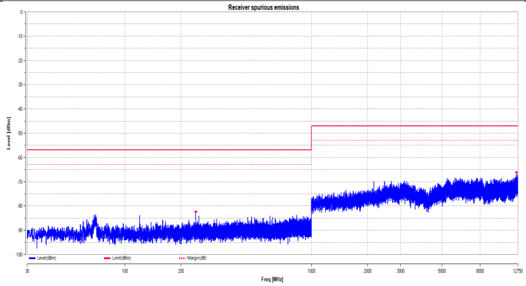
11N40SISO Ant1 2462
