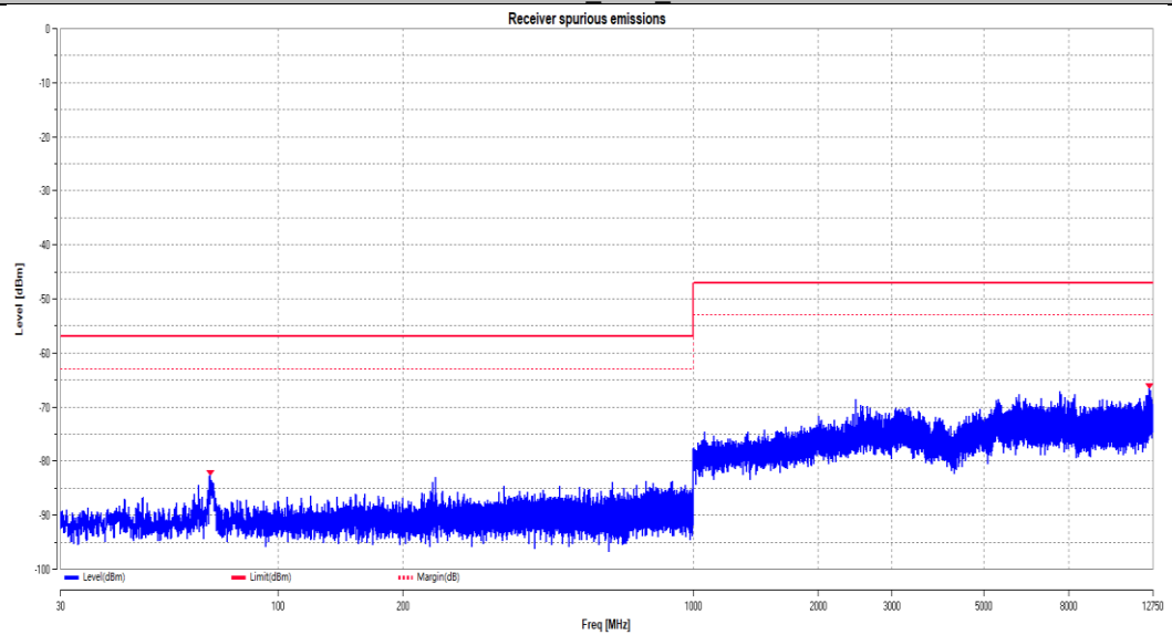
11N40SISO Ant1 2422
